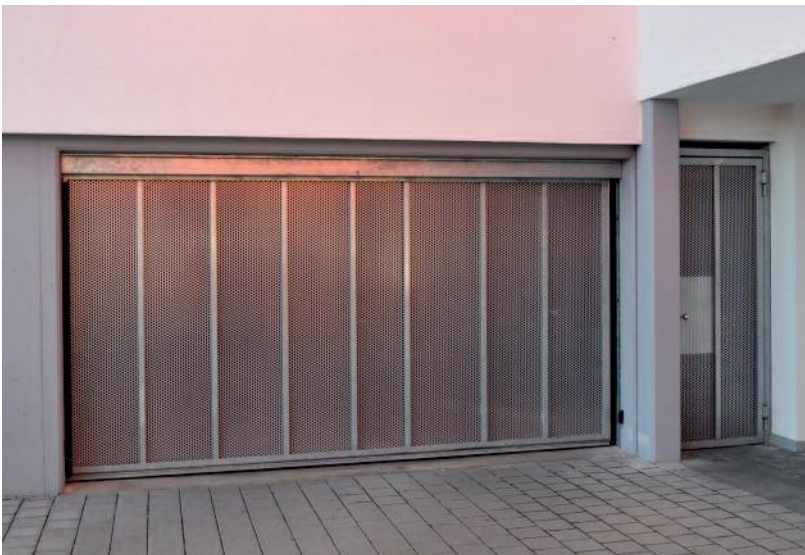
Verschleißarme Tor-Konstruktion für sehr hohe Bewegungszyklen
