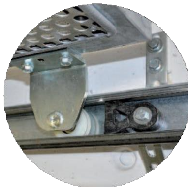
Kugelgelagerte Laufrollen sorgen jahrzehntlang für ruhigen und ausgeglichenen Torlauf
